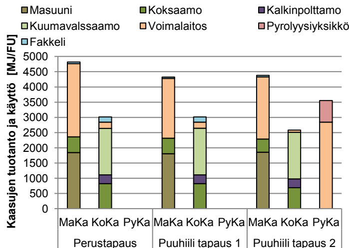
Kuva 3. Kolmen skenaarion kaasujen tuotto ja käyttö.
