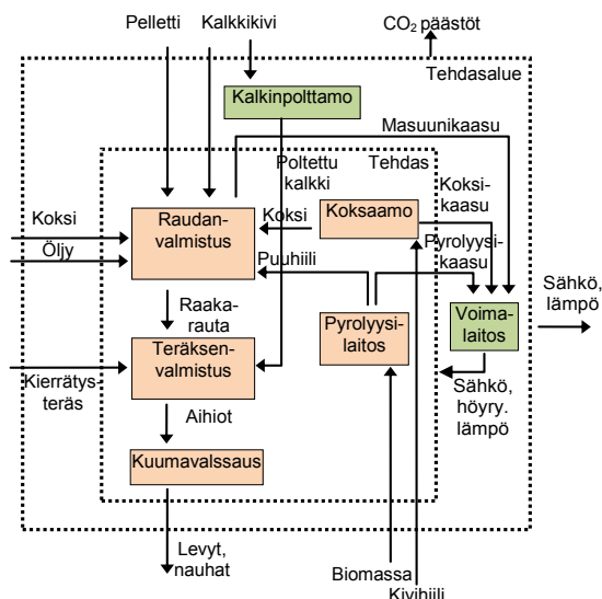
Kuva 2. Integroidun terästehtaan systeimirajaus.
